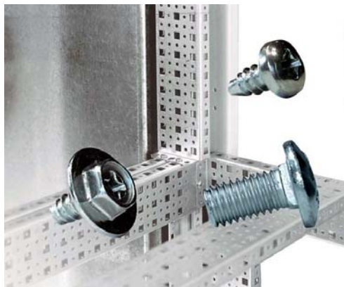
Foto: Schnell, stabil, hoch belastbar: Spezialschrauben für die Schaltschrankmontage von Lohmeier.
